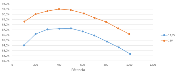
Rendimento % - 1000W-12E127S X Potência de saída
