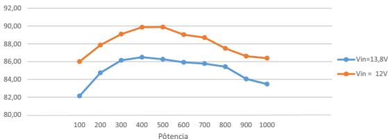
Rendimento % - 1000W-12E220S X Potência de saída
